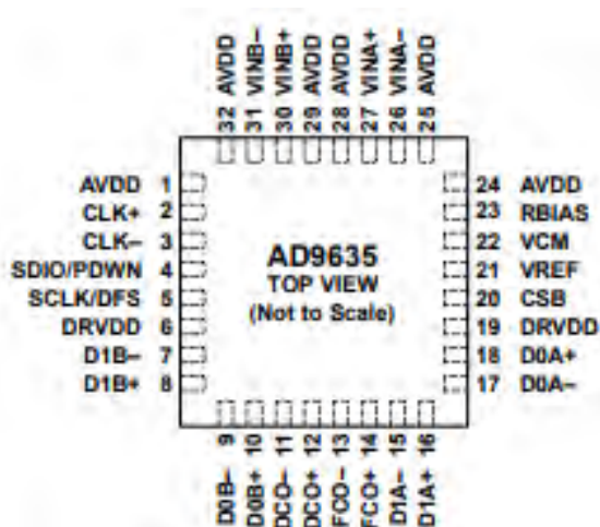
Рис.3.10. AD9635
