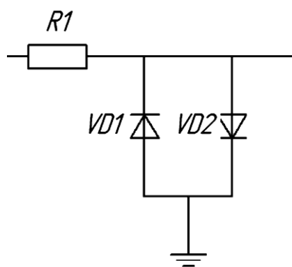
Рис. 3.4. Діодний обмежувач
