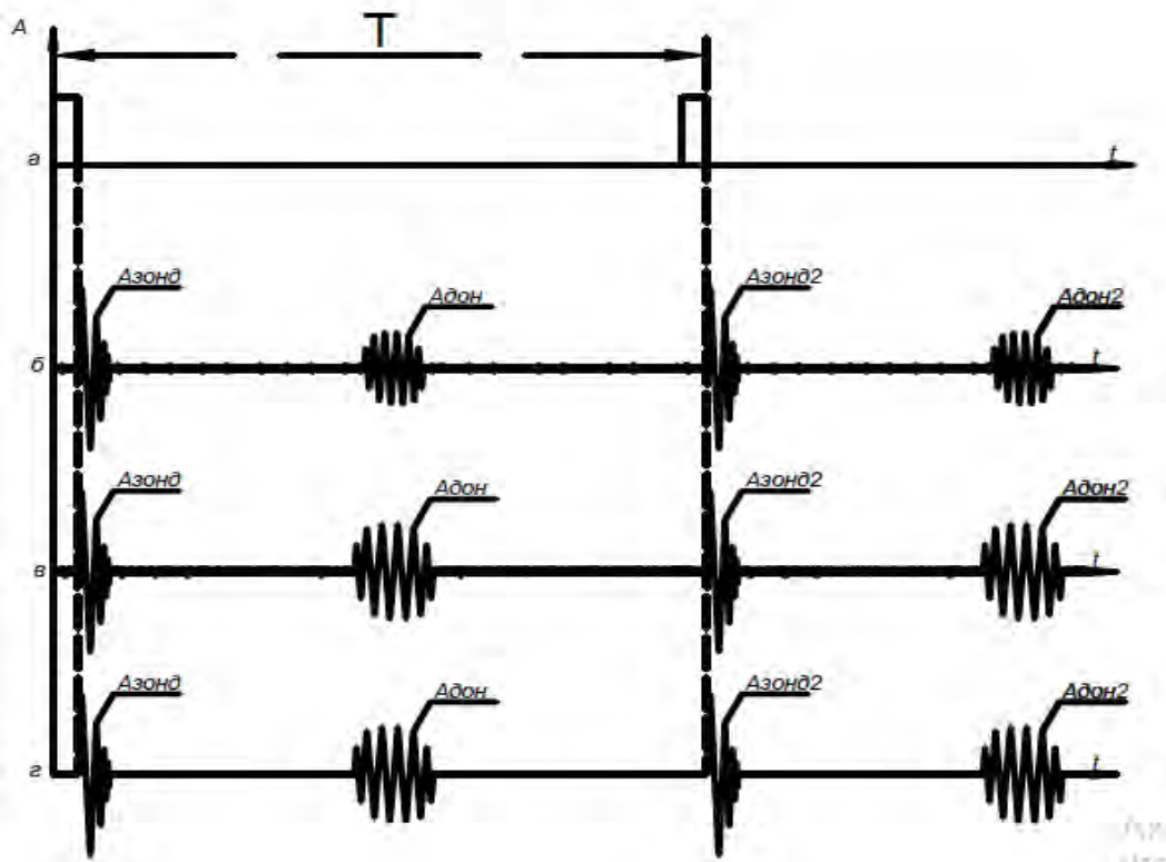
Рис.3.2.Часова діаграма
