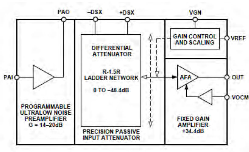
Рис.3.7. Функціональна блок-діаграма AD604
